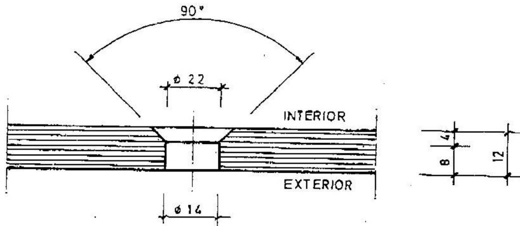
DETALLE TALADRO AVELLANADO
