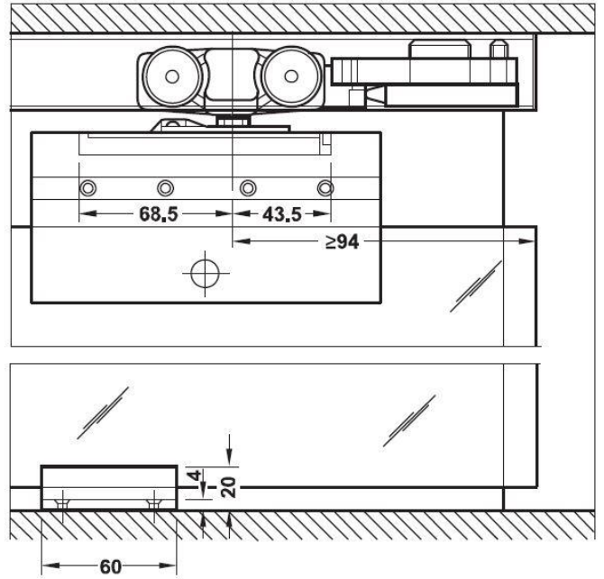
Corte del carrillo de traslación y guía
